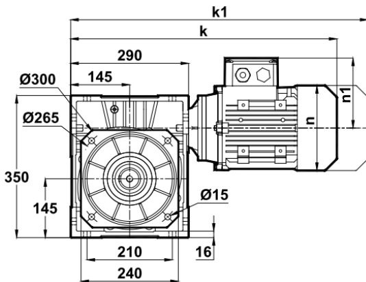
Размеры «к1» для электродвигателей с тормозом.
